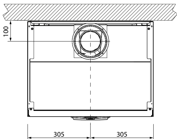
рис. 81- Вид сверху
