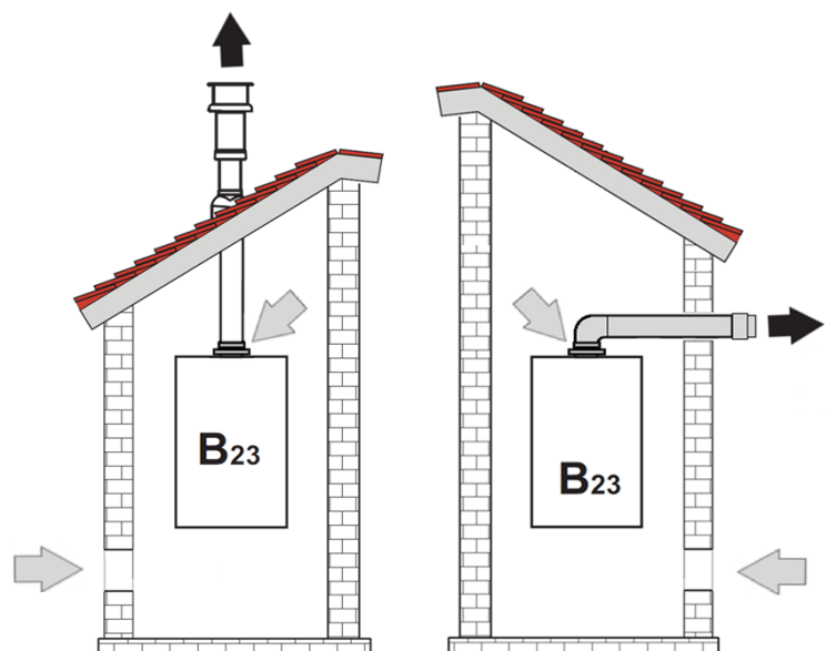
рис. 61- Примеры подключения
