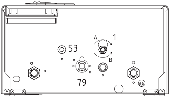
Рис. 2. Клапан наполнения
