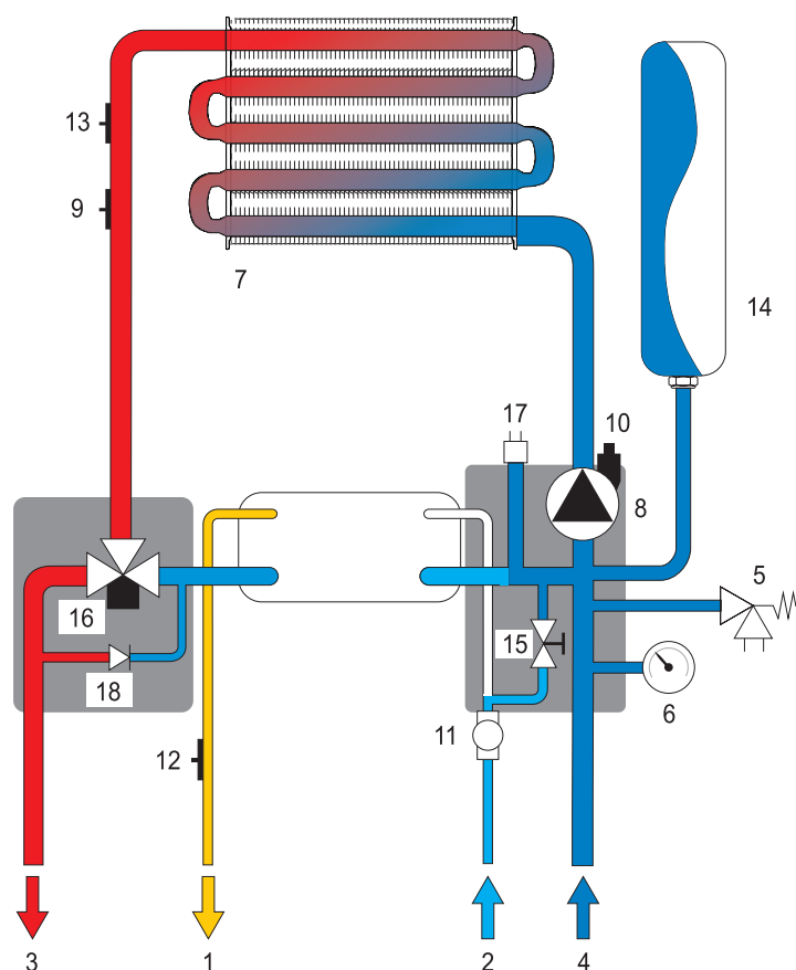
Рис. 14. Гидравлическая схема
