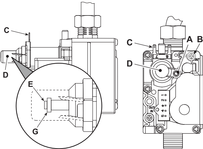
Рис. 14. Газовый клапан
