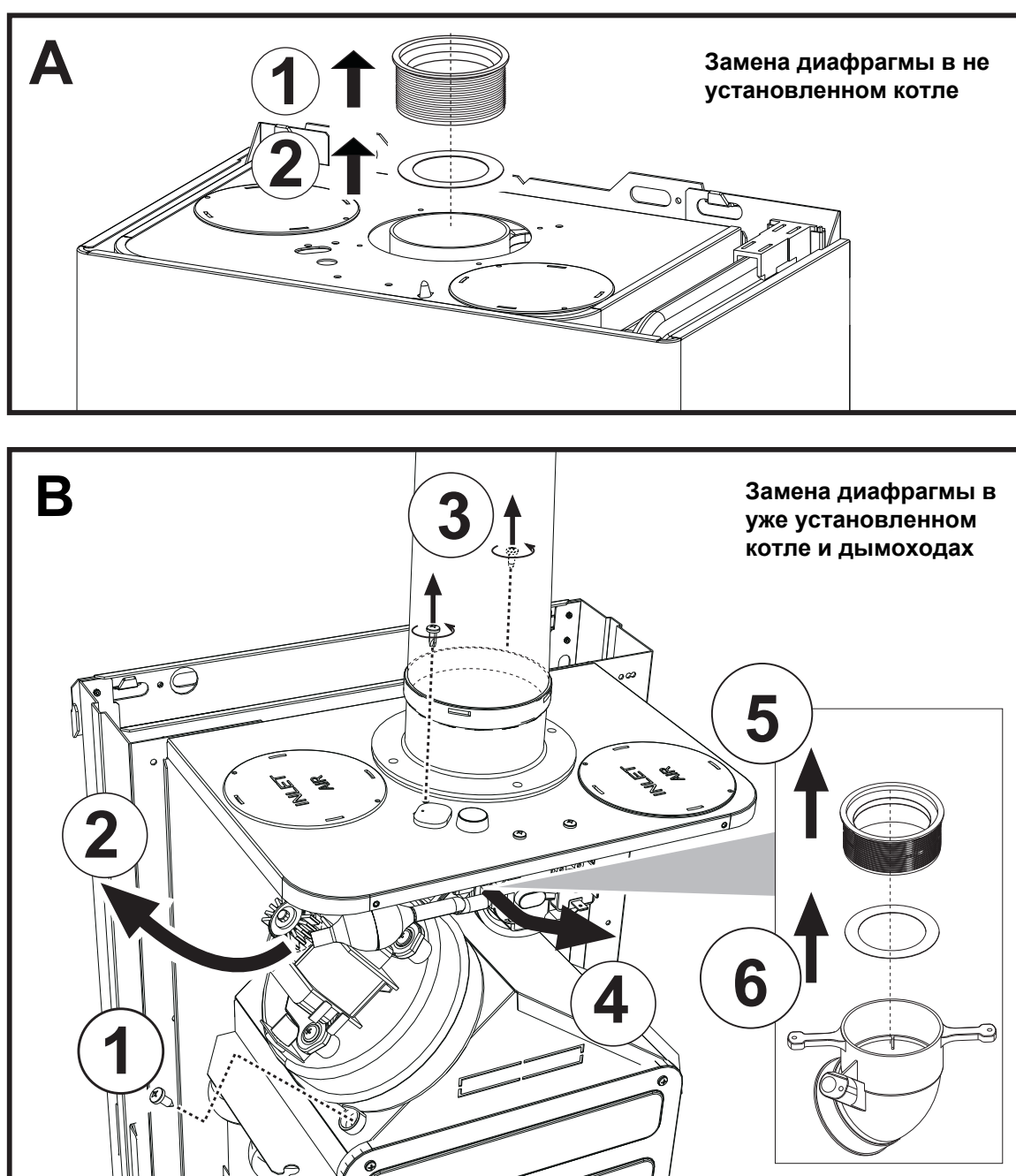
Рис. 28- Замена диафрагмы
