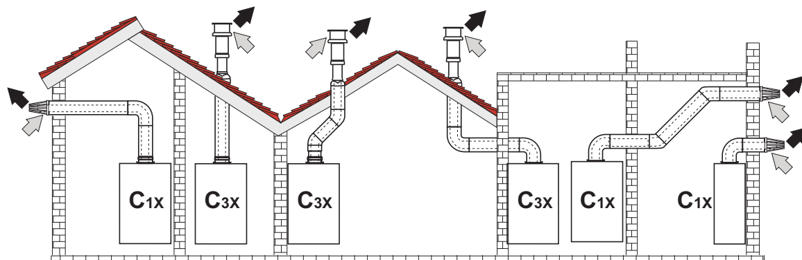
Рис. 29- Примеры подсоединения с помощью коаксиальных труб (→ = Воздух/ → = Дымовые газы)
