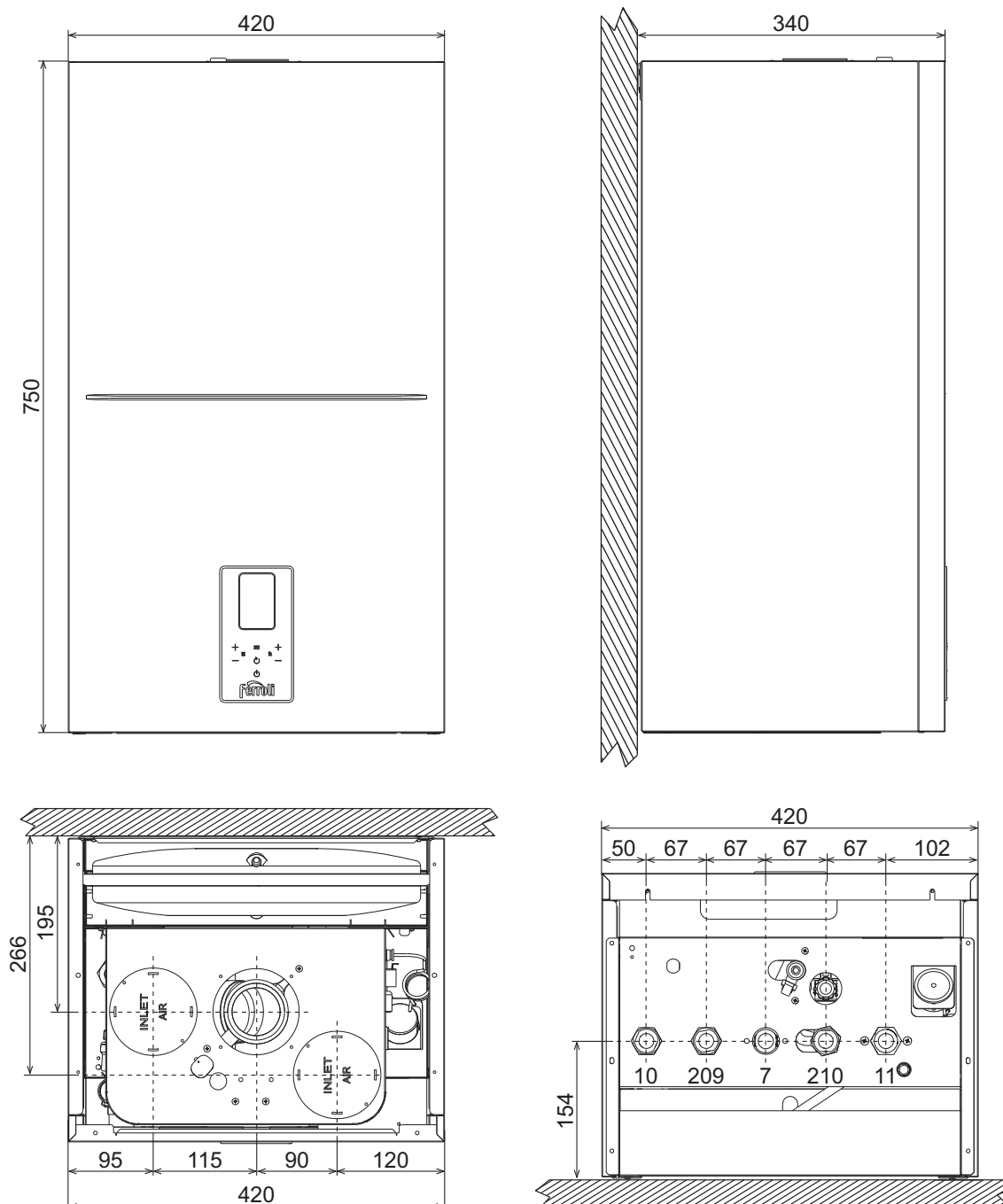
Рис. 41- Размеры и соединения модели DIVATOP D HF24
