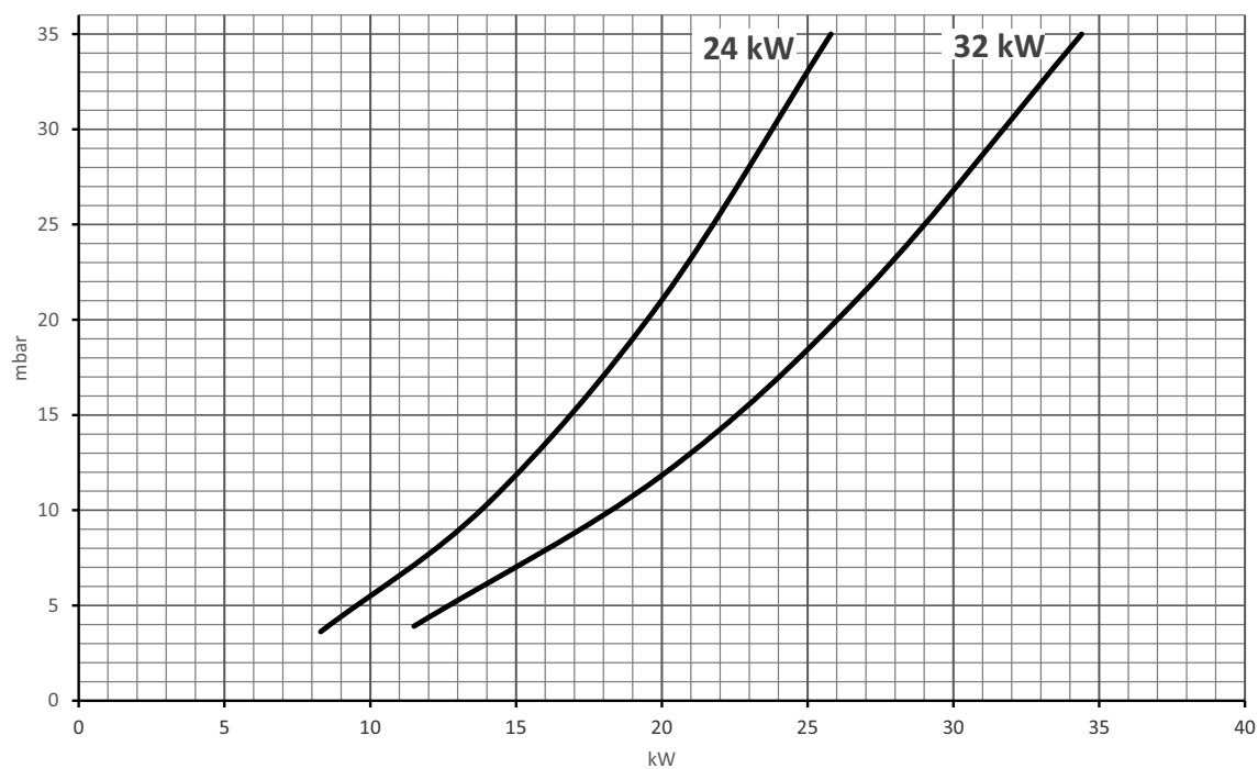
рис. 47- Диаграмма для версий, работающих на СНГ
