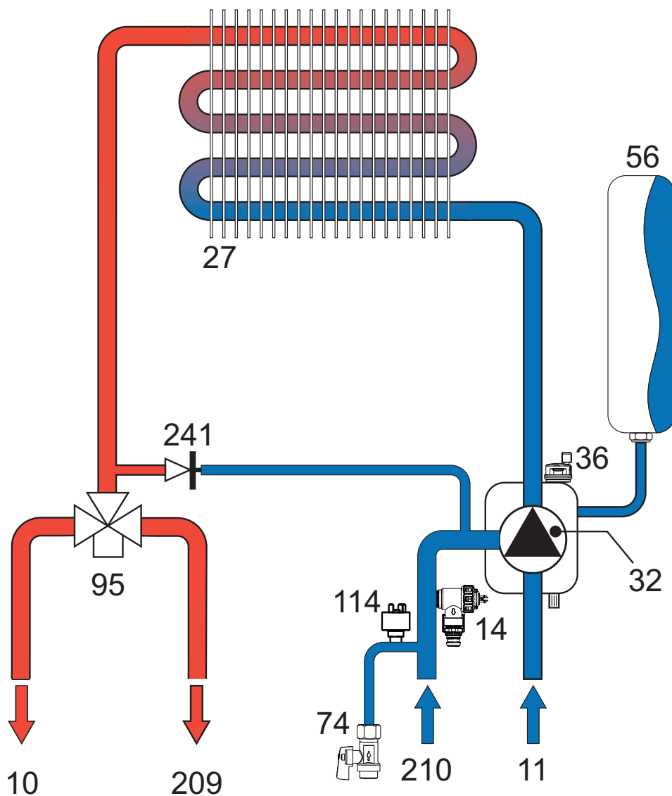
Рис. 45- Контур отопления
