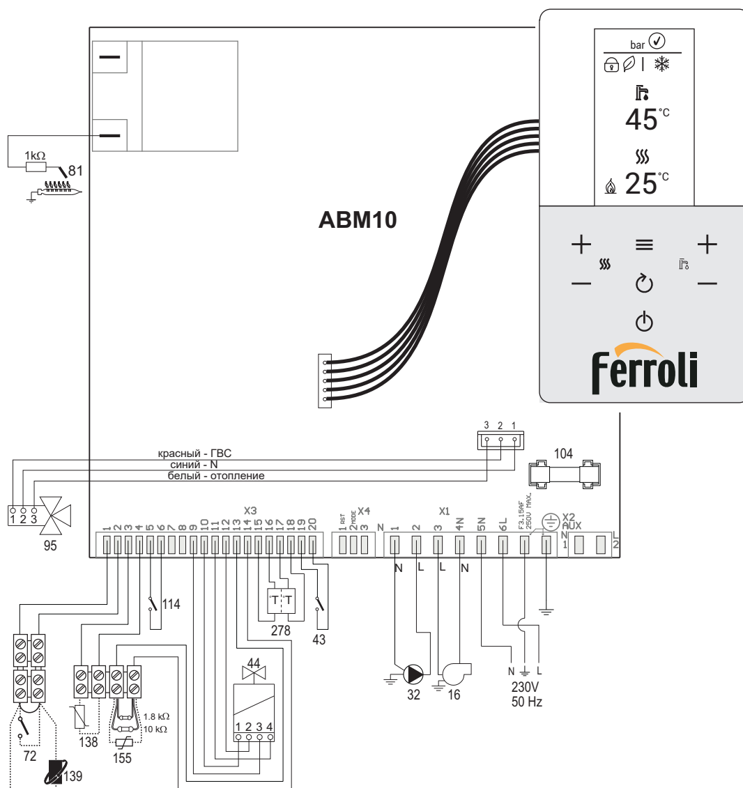
Рис. 48- Электрическая схема
