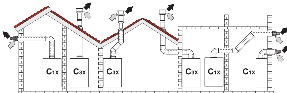
рис. 27- Примеры подсоединения с помощью коаксиальных труб (⇨ = Воздух/ ⇨ = Дымовые газы)
