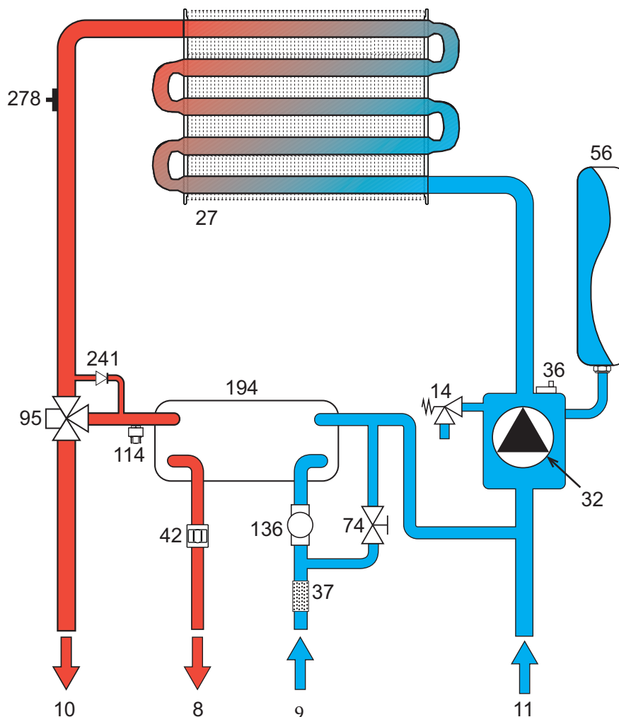
Рис. 36- Гидравлическая схема
