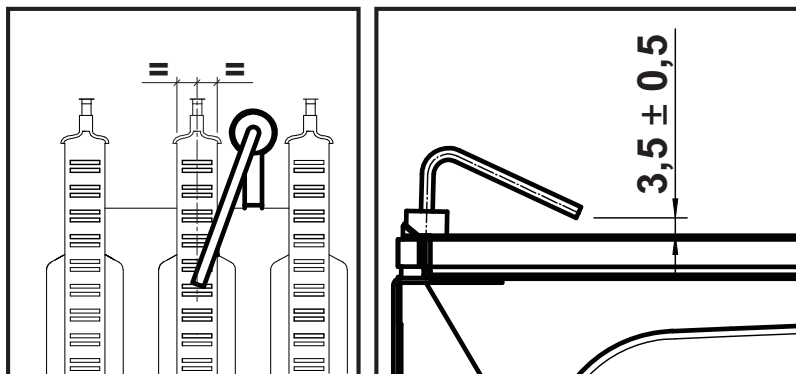
Рис. 32- Расположение электрода
