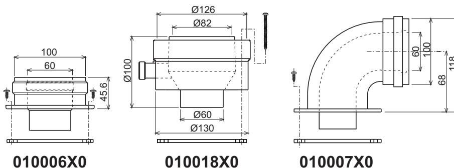
рис. 28- Исходные принадлежности для коаксиальных труб
