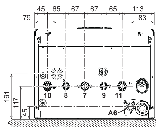
рис. 60- Вид снизу
