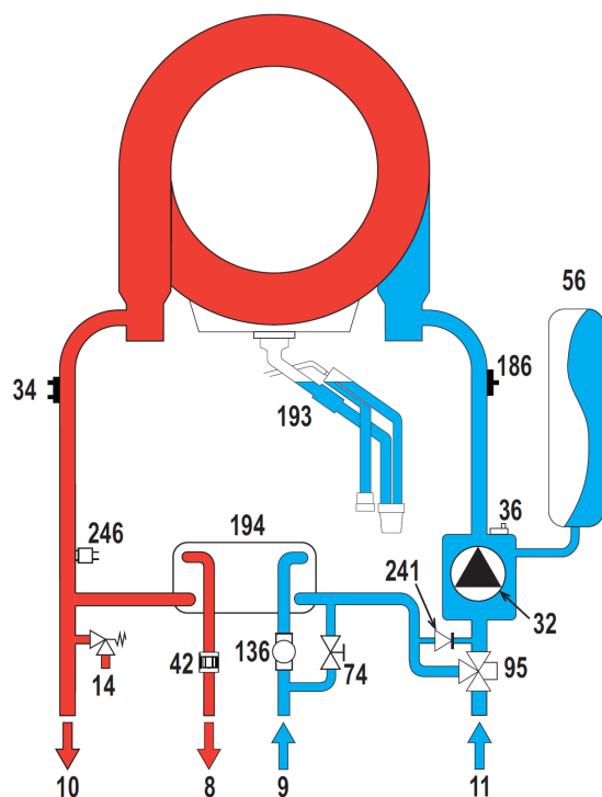
рис. 62- Гидравлический контур
