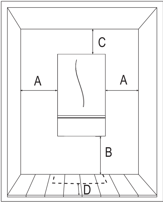
Рис. 7. Размещение котла
