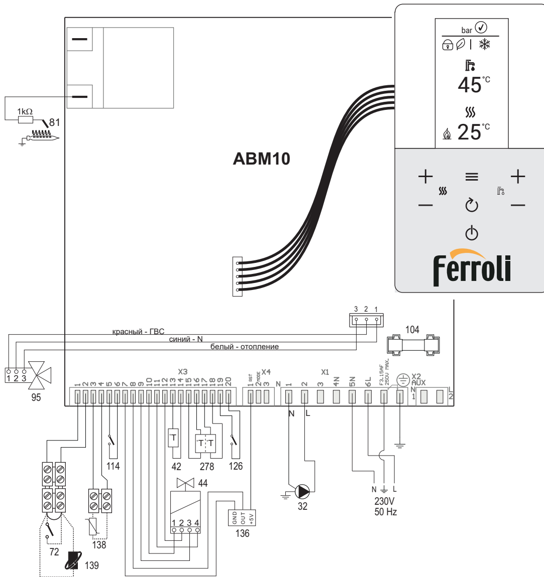
рис. 39- Электрическая схема
