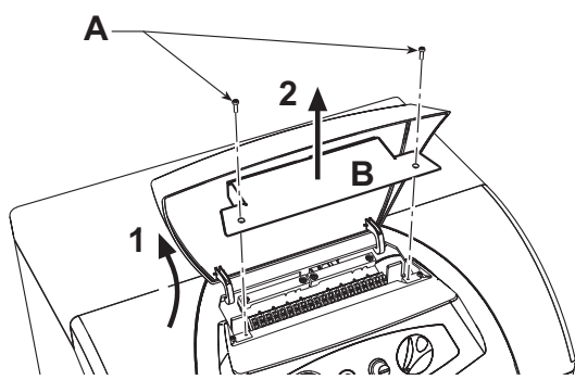
ΕΙΚ. 4 - Πρόσβαση στη βάση ακροδεκτών
