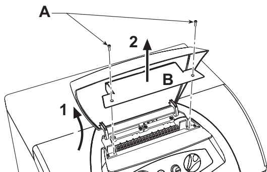
fig. 4 - Accesso alla morsettiere
