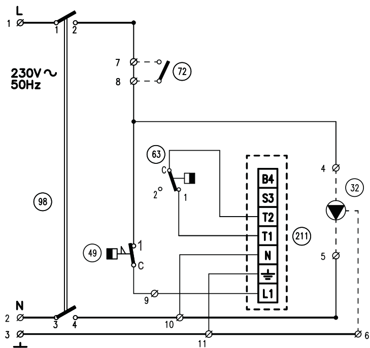
fig. 7 - Elektrisch blokschema ATLAS 32-78
