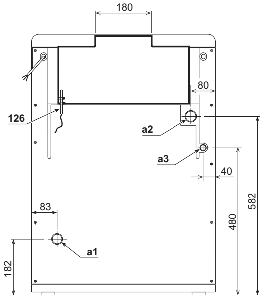
рис. 11 - Вид сзади
