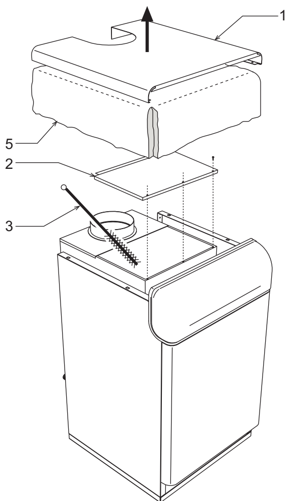
рис. 5 - Очистка котла
