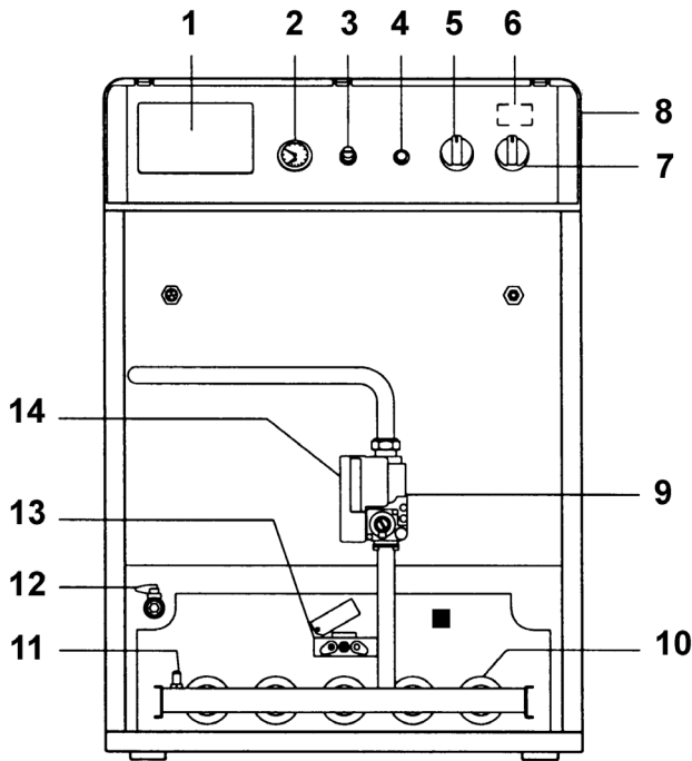
рис. 12 - Общий вид
