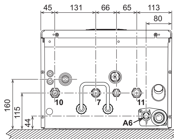
рис. 51- Вид снизу
