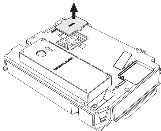
рис. 47- Посадочное место предохранителя
