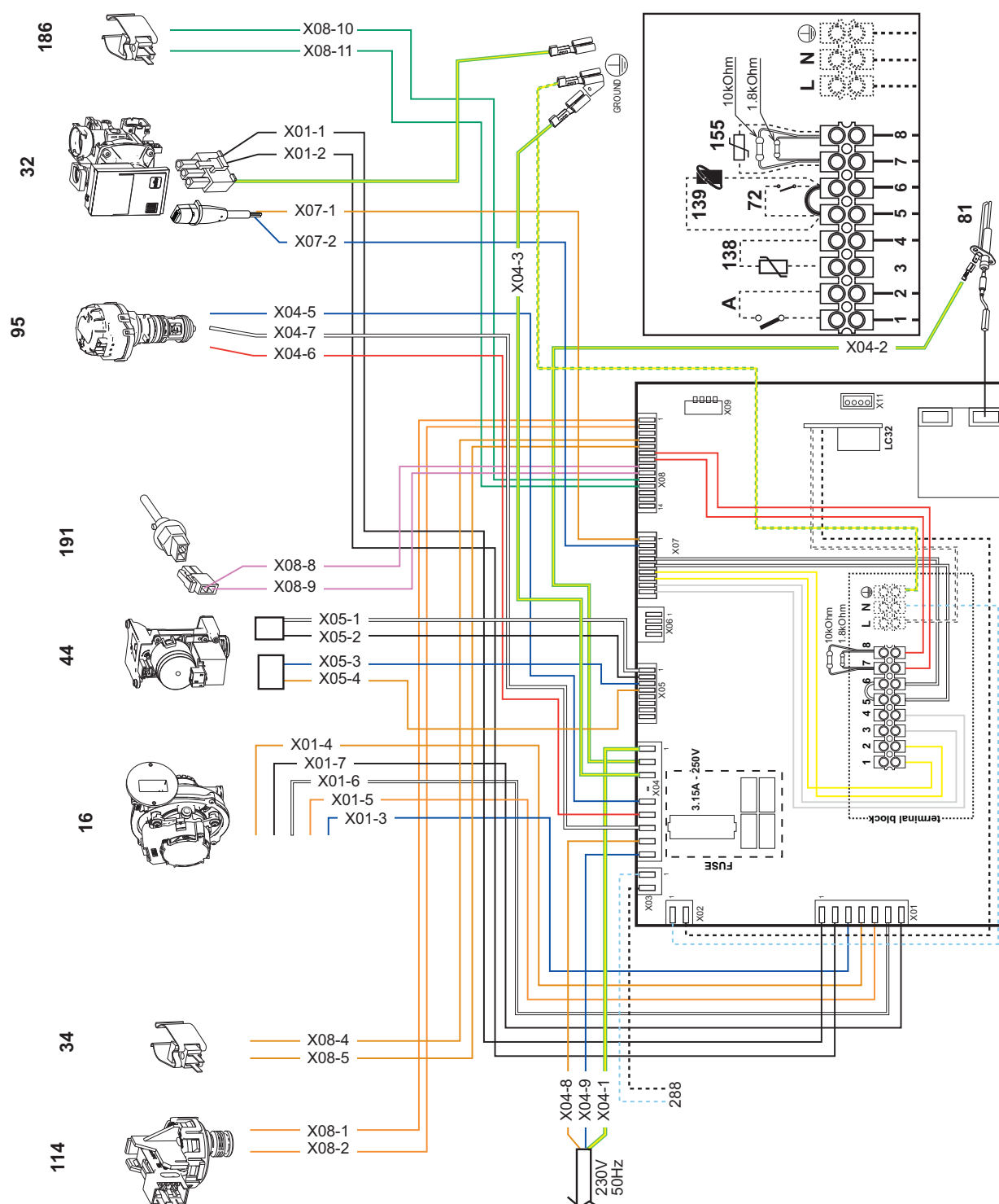
рис. 57- Электрическая схема
