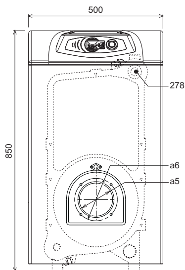
fig. 19 - Vista anteriore
