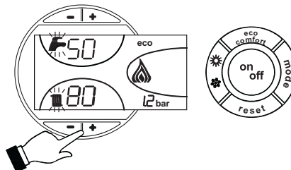
fig. 18 - Modalità TEST
