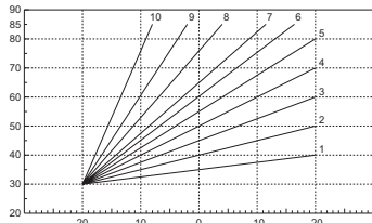
рис. 14 - Компенсационные характеристики
