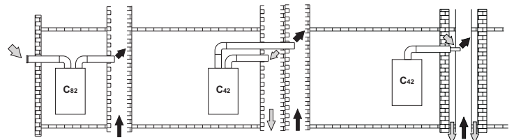
рис. 25 - Примеры подсоединения к дымоходам (⇨ = Воздух / ⇨ = Продукты сгорания)
