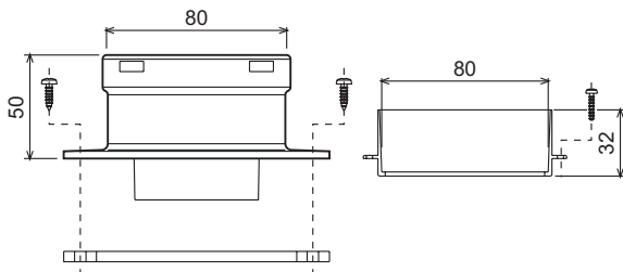
рис. 24 - Соединительный элемент для раздельных труб
