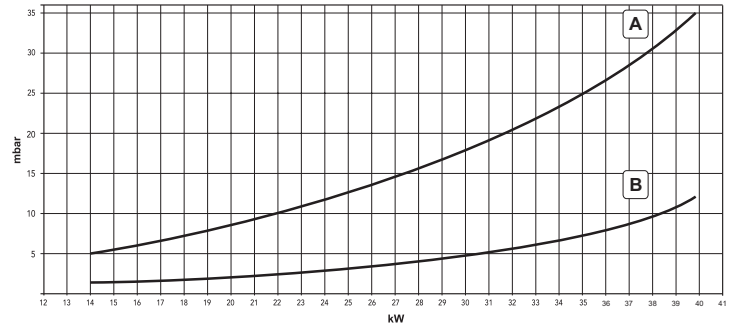
рис. 37 - Диаграммы давление - мощность DIVAtop MICRO F 37
