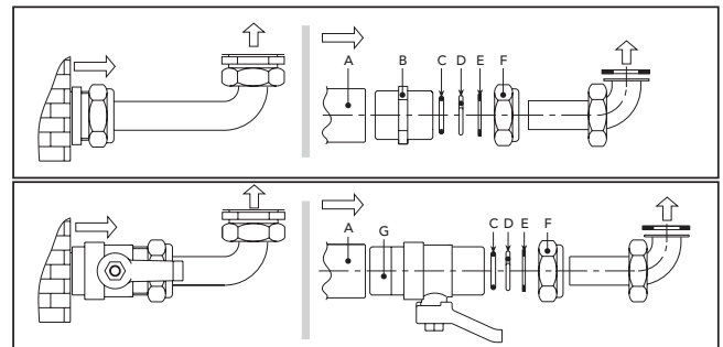
рис. 18 - Соединительный комплект
