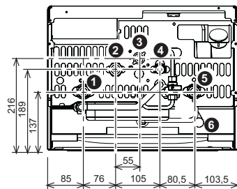
рис. 17 - Гидравлические соединения
