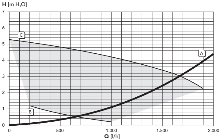
мал. 29 - Втрати напору / Напір циркуляційних насосівBLUEHELIX TECH 18/25
