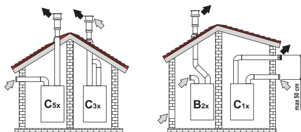
рис. 18 - Примеры подсоединения с помощью раздельных труб (→ = Воздух / → = дымовые газы)
