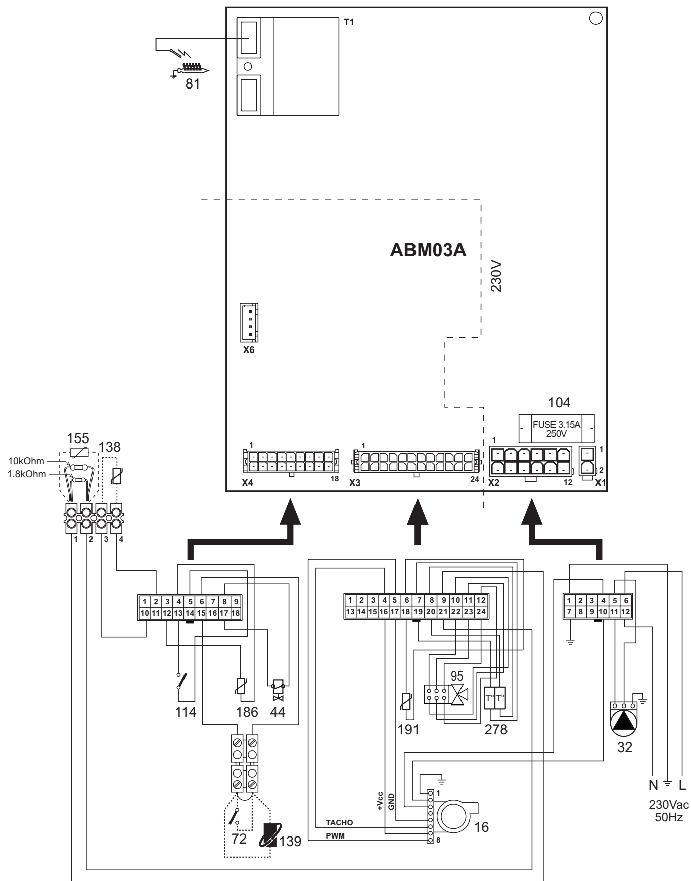
рис. 31 - Электрическая схема
