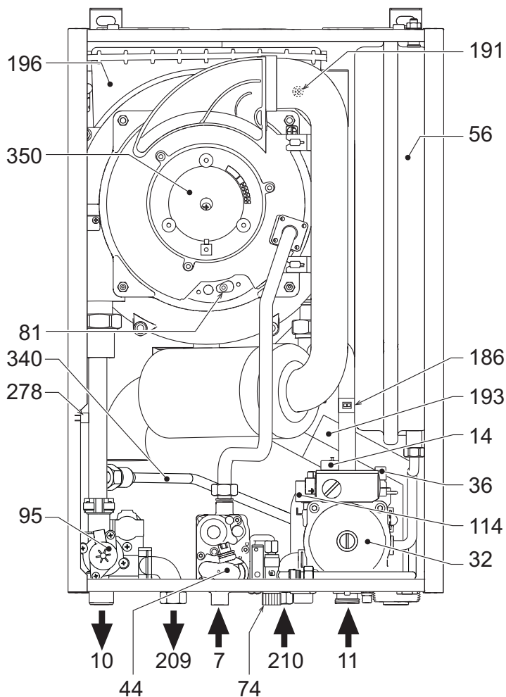
рис. 27 - Общий вид
