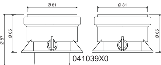
рис. 19 - Соединительный элемент для раздельных труб
