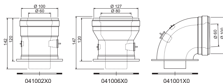
мал. 17 - Початкові елементи для коаксialьних трубопроводів
