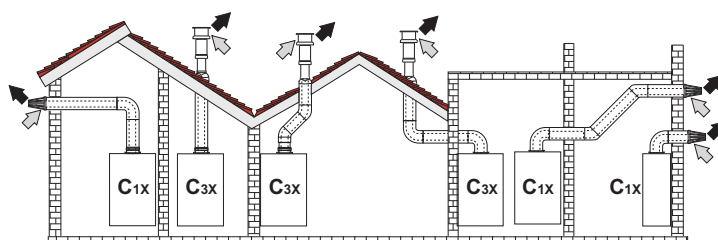
мал. 16 - Приклад підключення за допомогою співісних (коаксialьних) труб (⇐ = Повітря / ⇨ = Відпрацьовані гази)
