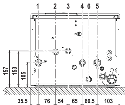
рис. 13 - Гидравлические штуцеры
