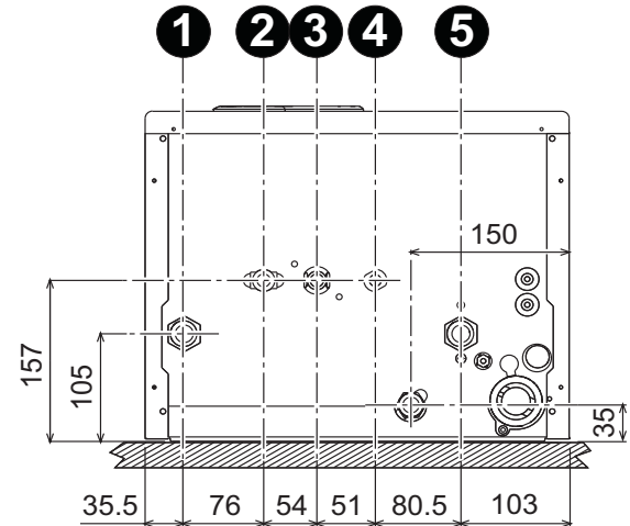
рис. 13 - Гидравлические штуцеры
