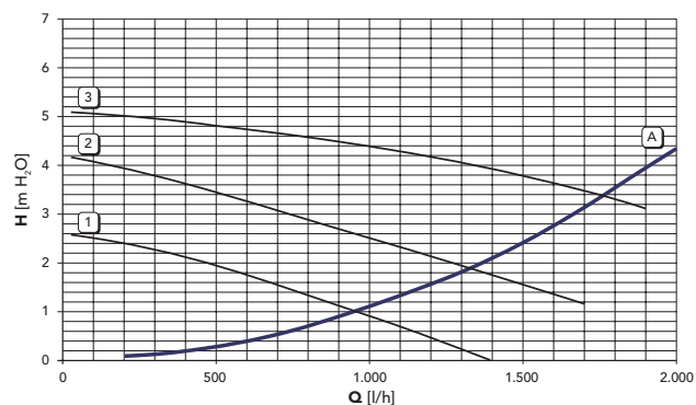
рис. 19 - Потери напора циркуляционных насосов DOMIproject F 24 D
