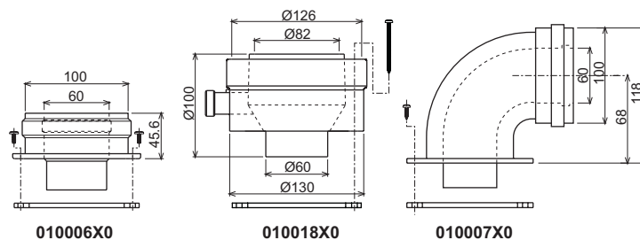
рис. 10 - Элементы для коаксиальных воздуховодов
