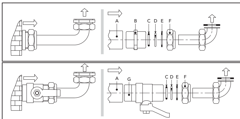
рис. 7 - Соединительный комплект
