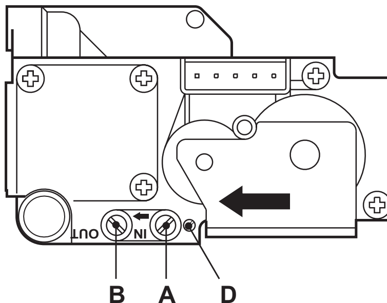
рис. 10 - Газовый клапан
