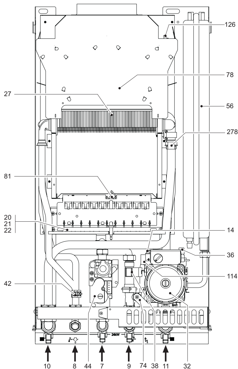
рис. 13 - Общий вид
