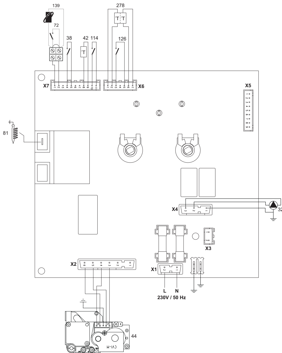
рис. 15 - Электрическая схема
