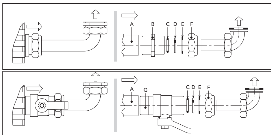
рис. 7 - Соединительный комплект
