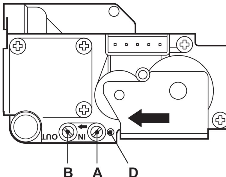
рис. 16 - Газовый клапан
