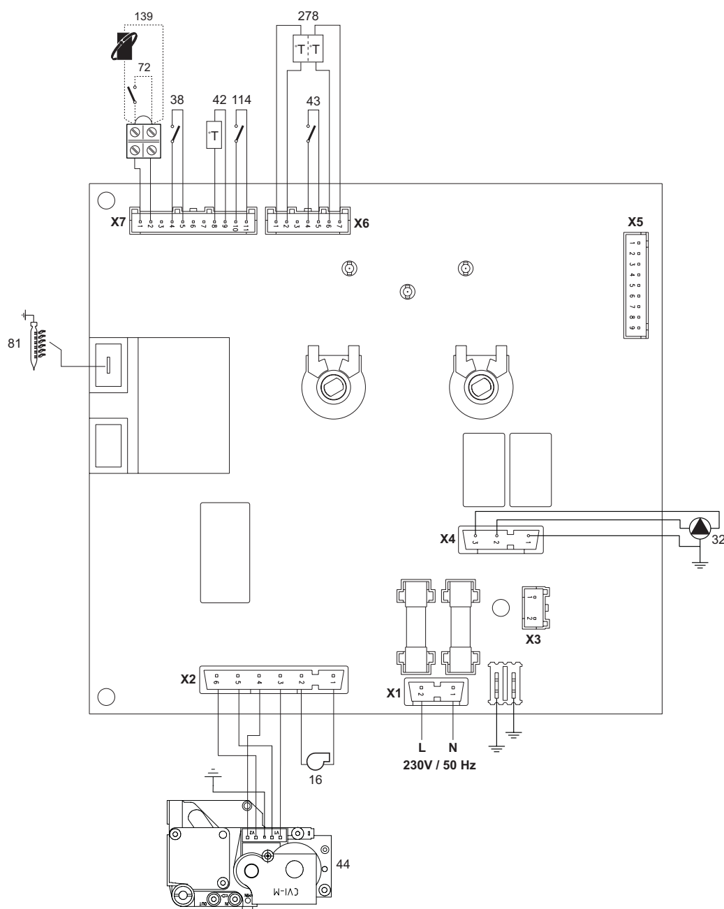
рис. 22 - Электрическая схема
