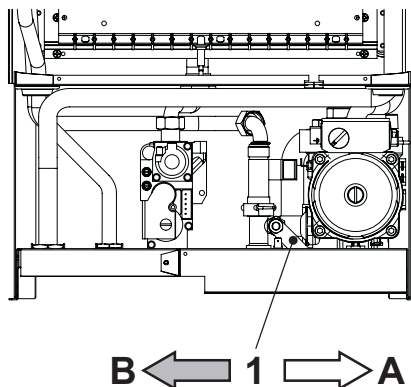
рис. 6 - Кран для заливки воды
