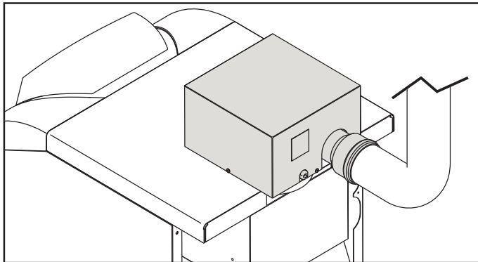
рис. 4 - Комплект дымососа
