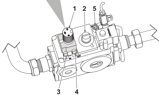
рис. 2 - Газовый клапан
