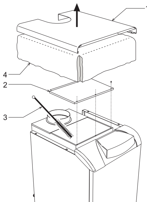
рис. 9 - Очистка котла
