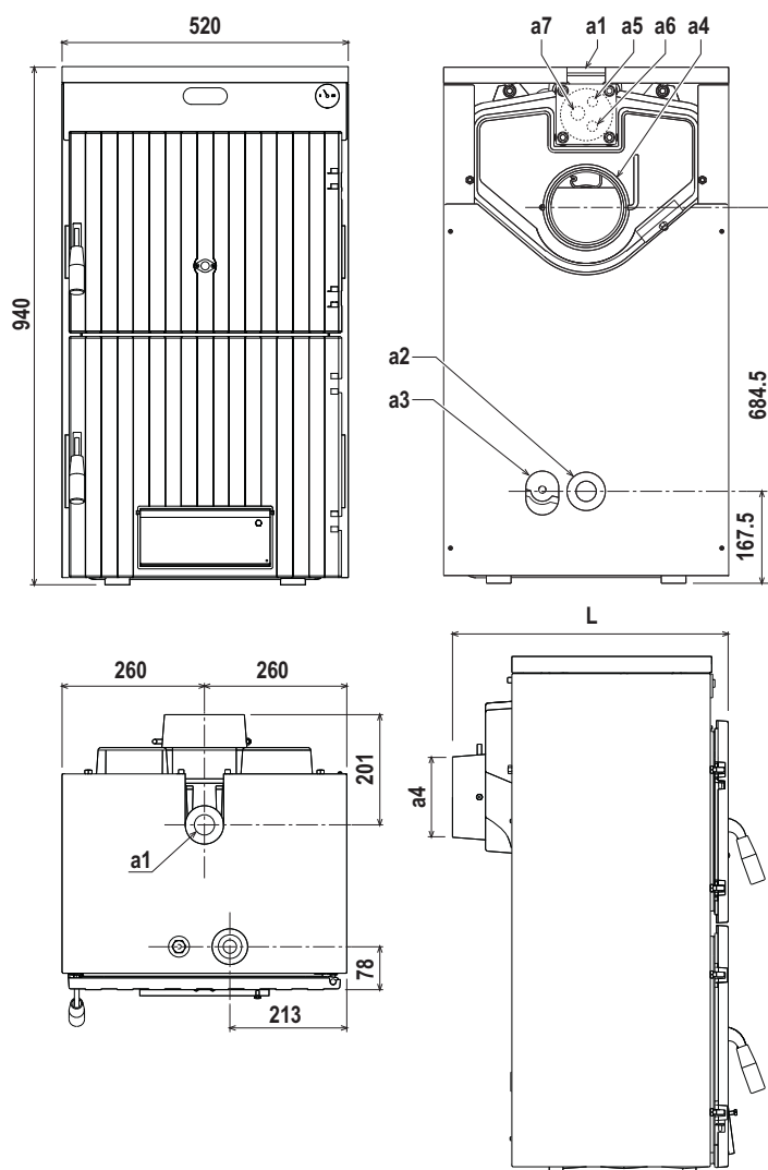
рис. 17 - Габаритные размеры и подключения
