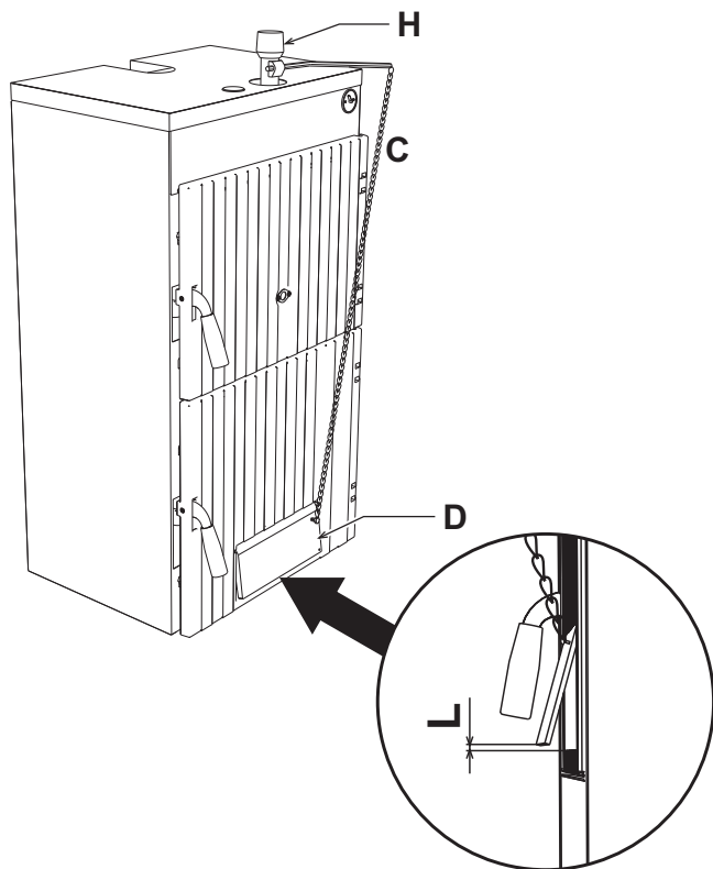
рис. 2 - Монтаж
