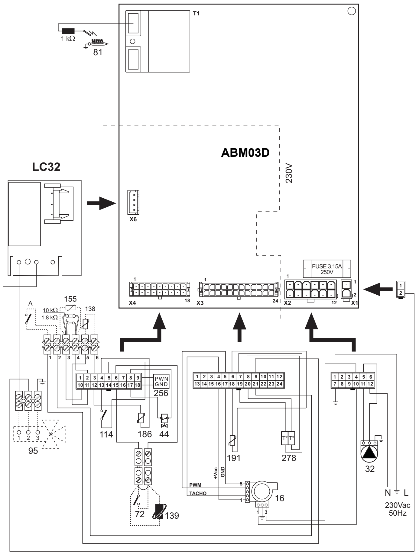
fig. 29 - Schemă electrică
