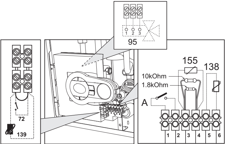
fig. 14 - Accesso alla morsettiere
