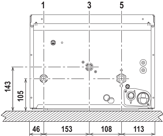
рис. 12 - Гидравлические соединения
