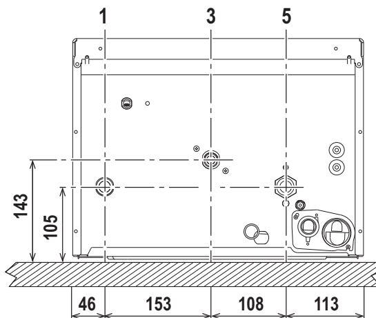
fig. 12 - Attacchi idraulici
