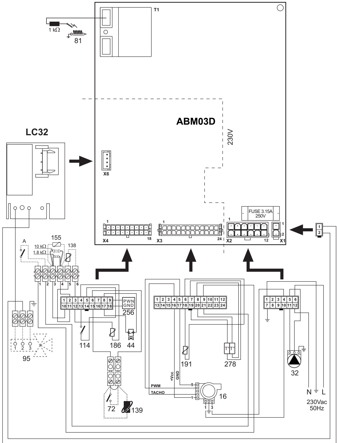
fig. 29 - Esquema eléctrico
