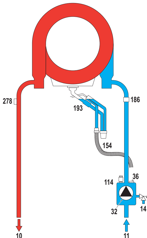
мал. 28 - Гідравлічний контур
