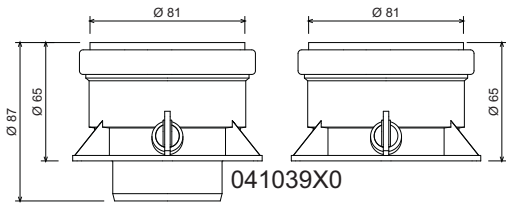
рис. 18 - Соединительный элемент для раздельных труб
