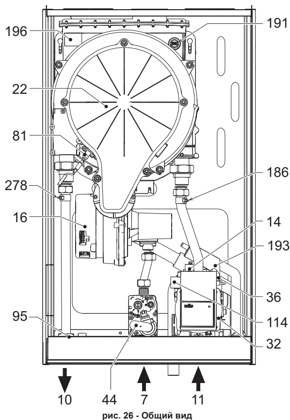
рис. 26 - Общий вид
