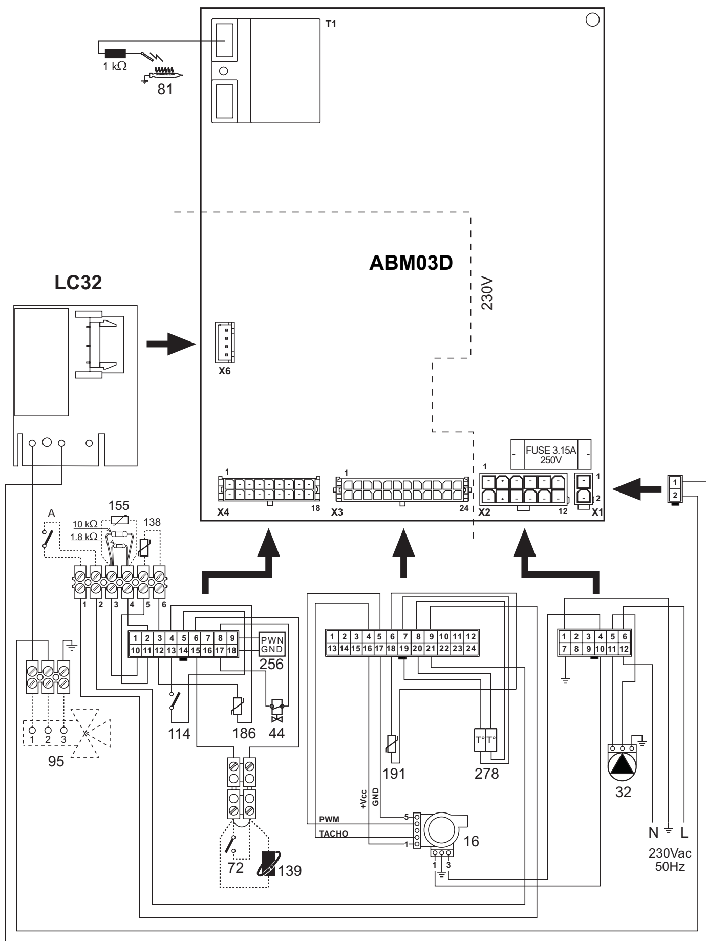
fig. 29 - Schema elettrico
