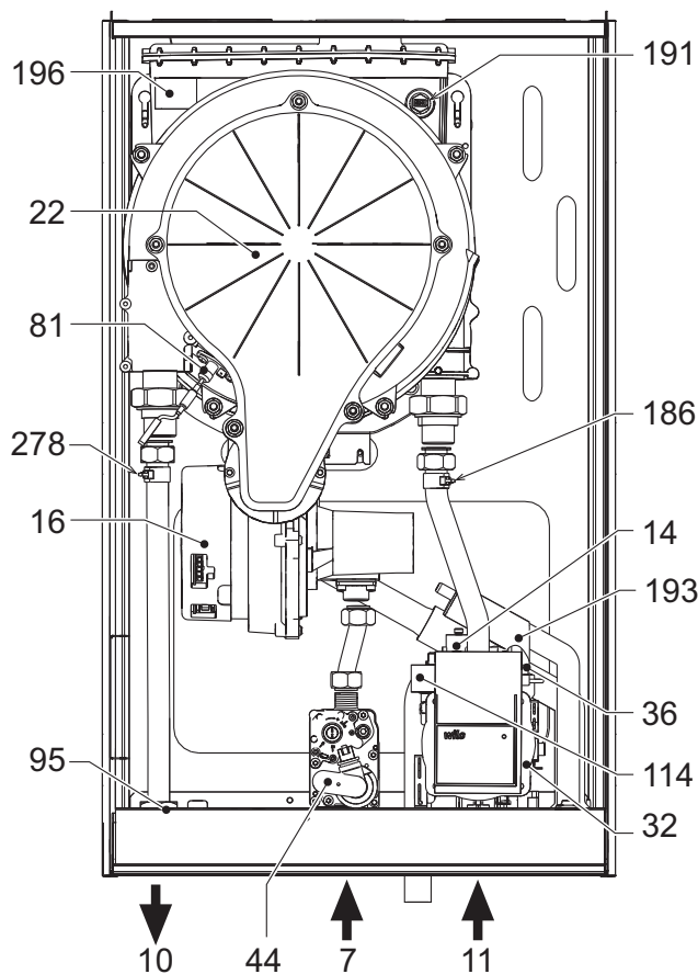
fig. 26 - Vista generale
