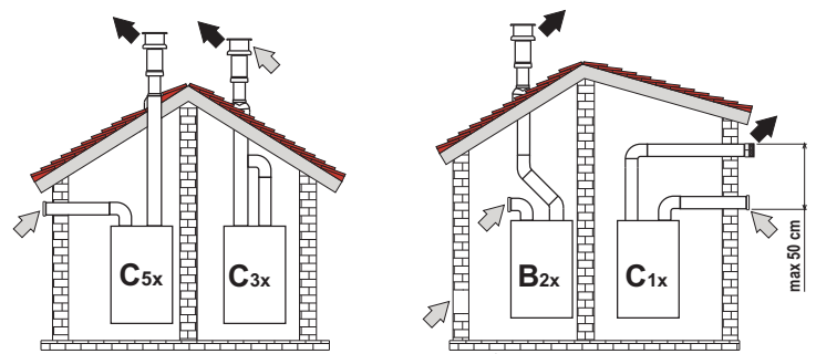
şek. 17 - Aynı borularla bağlantıya örnek (→ = Hava / → = Duman)
