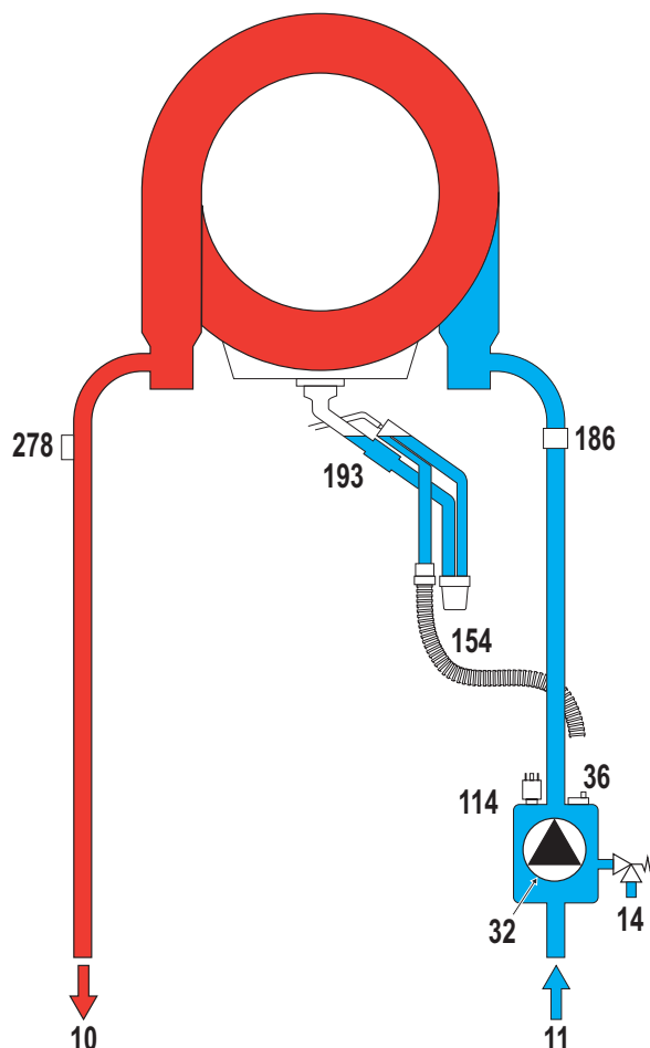
fig. 28 - Circuitul hidraulic
