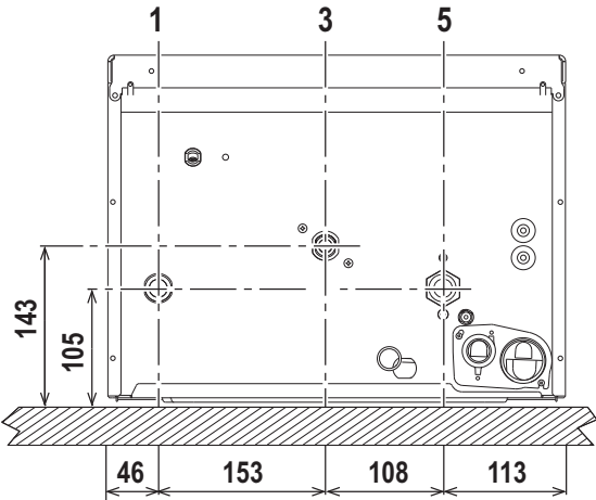
fig. 12 - Conexiones hidráulicas
