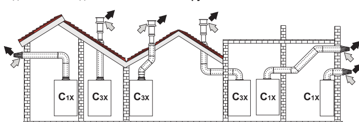
мал. 15 - Приклад підключення за допомогою співвісних (коаксіальних) труб (→ = Повітря / → = Відпрацьовані гази)
