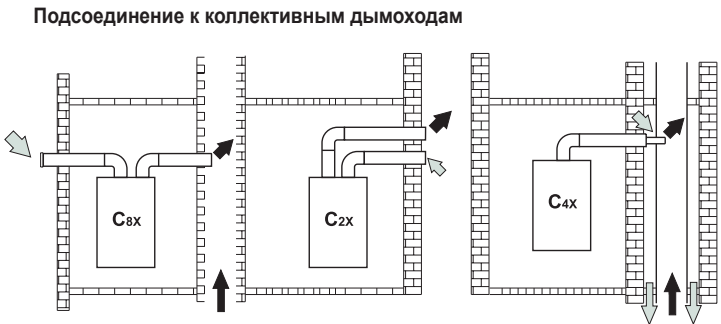
Рис. 14. Примеры подсоединения к дымоходам ⇨ – воздух; ⇨ – дымовые газы
