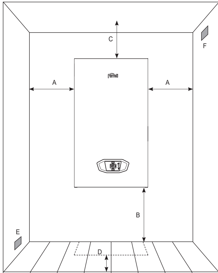
Рис. 3. Место установки
