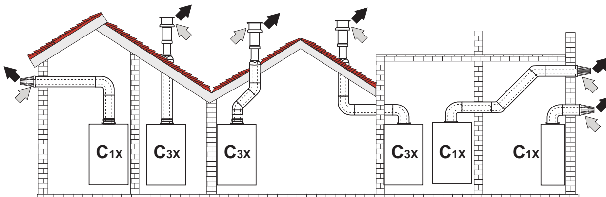
Рис. 12- Примеры подсоединения с помощью коаксиальных труб (⇨ = Воздух/ ⇨ = Дымовые газы)
