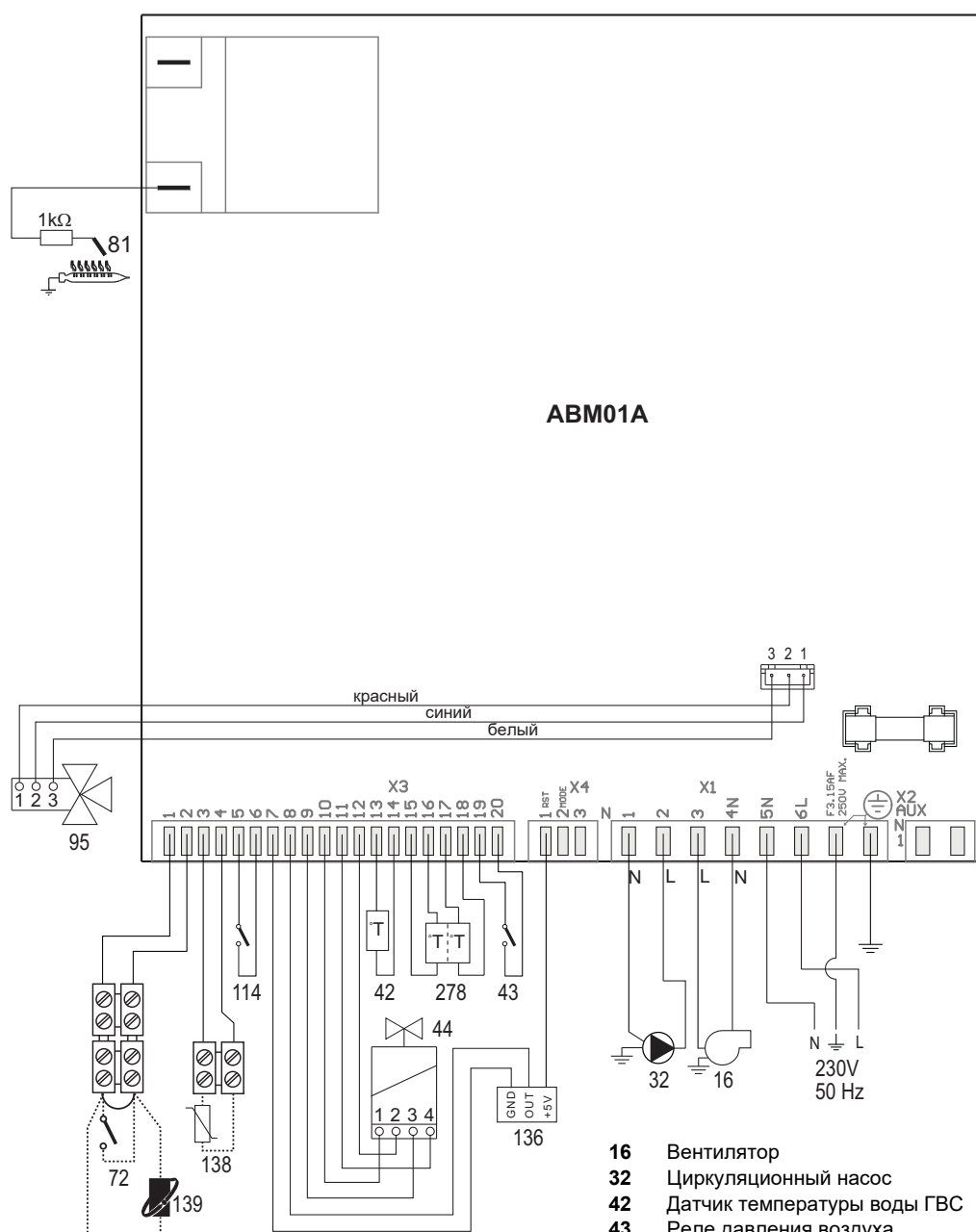
Рис. 28- Электрическая схема
