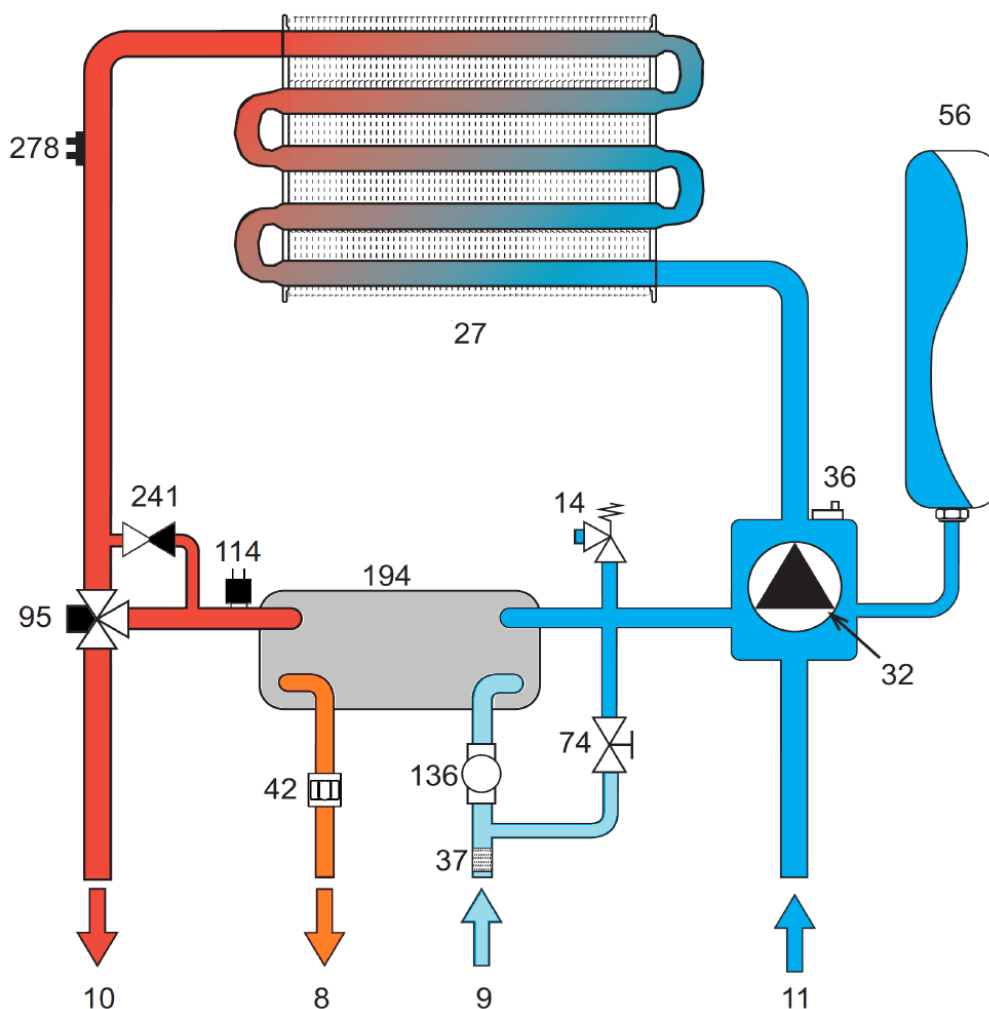
Рис. 27 - Гидравлическая схема Diva D F
