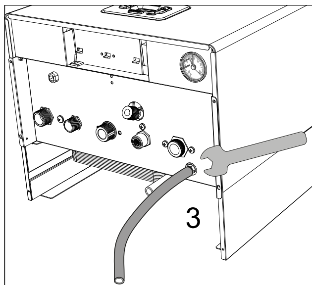
Рис. 9 - Кран слива
