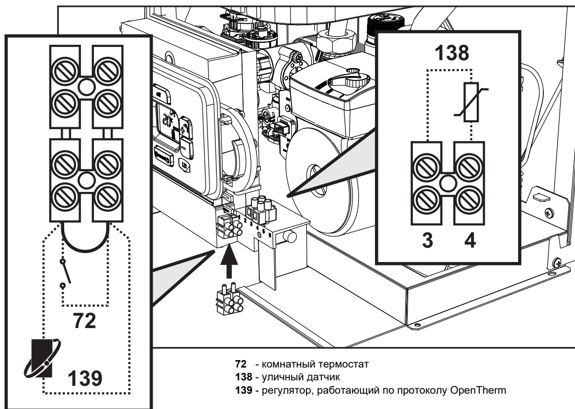
Рис. 10 - Доступ к клеммной колодке
