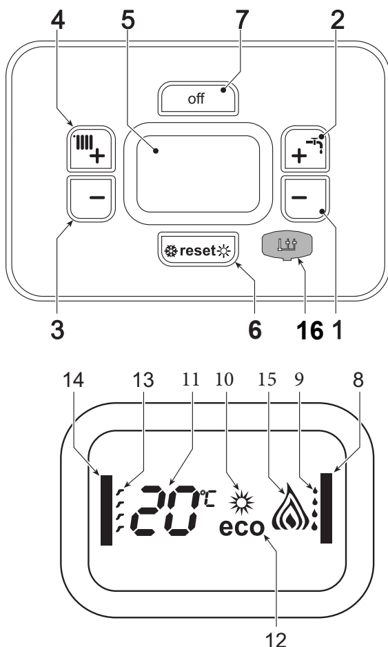
Рис. 1- Панель управления
