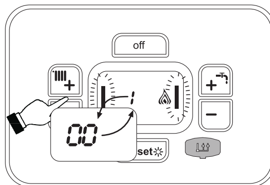
Рис. 17 - Режим «TEST» (мощность системы отопления = 100%)
