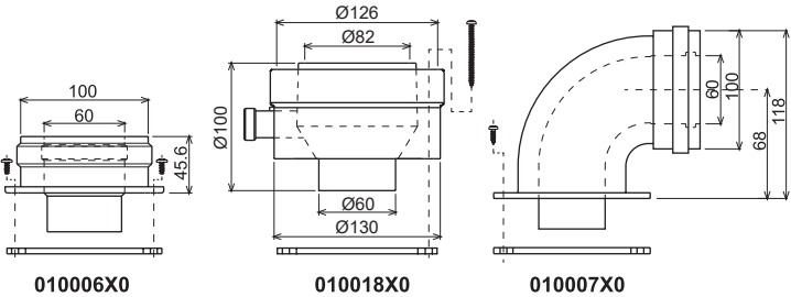
Рис. 9. Начальные элементы для коаксиальных дымоходов
