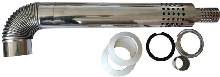
Рис 9А. Коаксиальный дымоход 80/127 (арт. 902601230)
