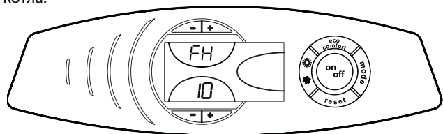
рис. 5 - Включение котла
